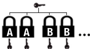
Cadenas s'entreouvrant sur clé passe MK-KA (MasterKeyed Keyed-Alike)
