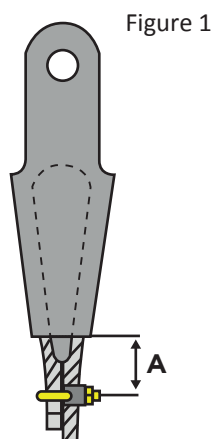
Serre-câble selon la norme EN 13411-5
